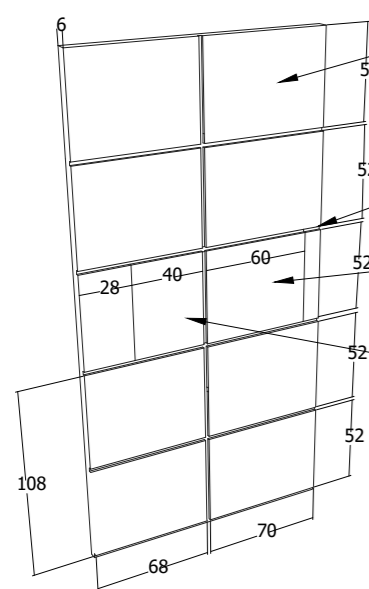
PAINEL DG DADOS E ELÉTRICO SEM ESCALA
